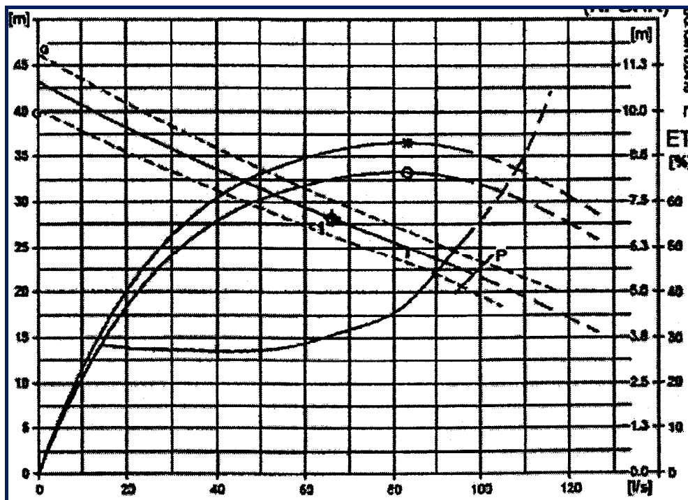
Diagramma 01 – Caratteristiche di funzionamento
